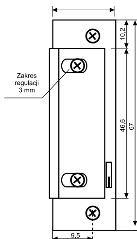
Elektrozaczepty radialny serii 1400 RF
