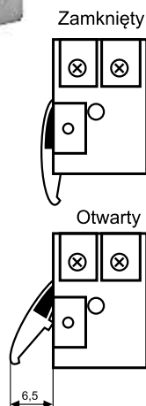
Elektrozaczepty tradycyjny serii 1400
